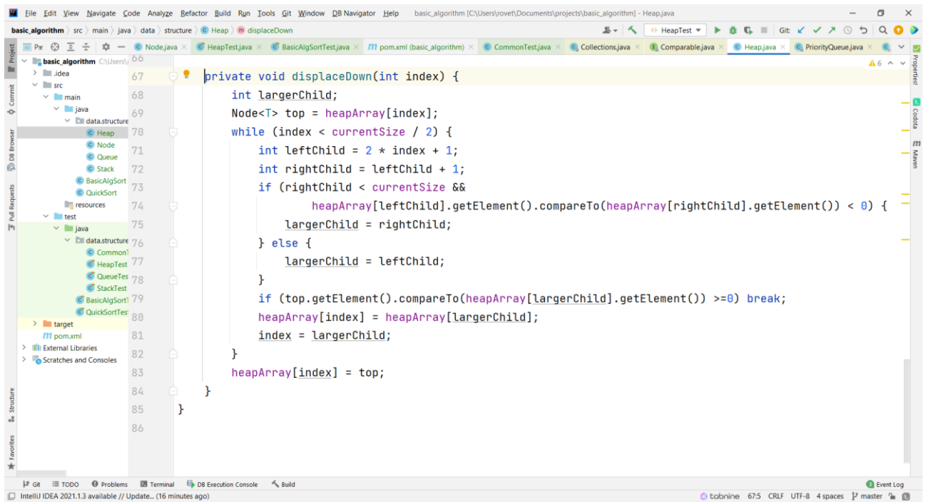
Рис.1. Реалізація структури даних піраміди
