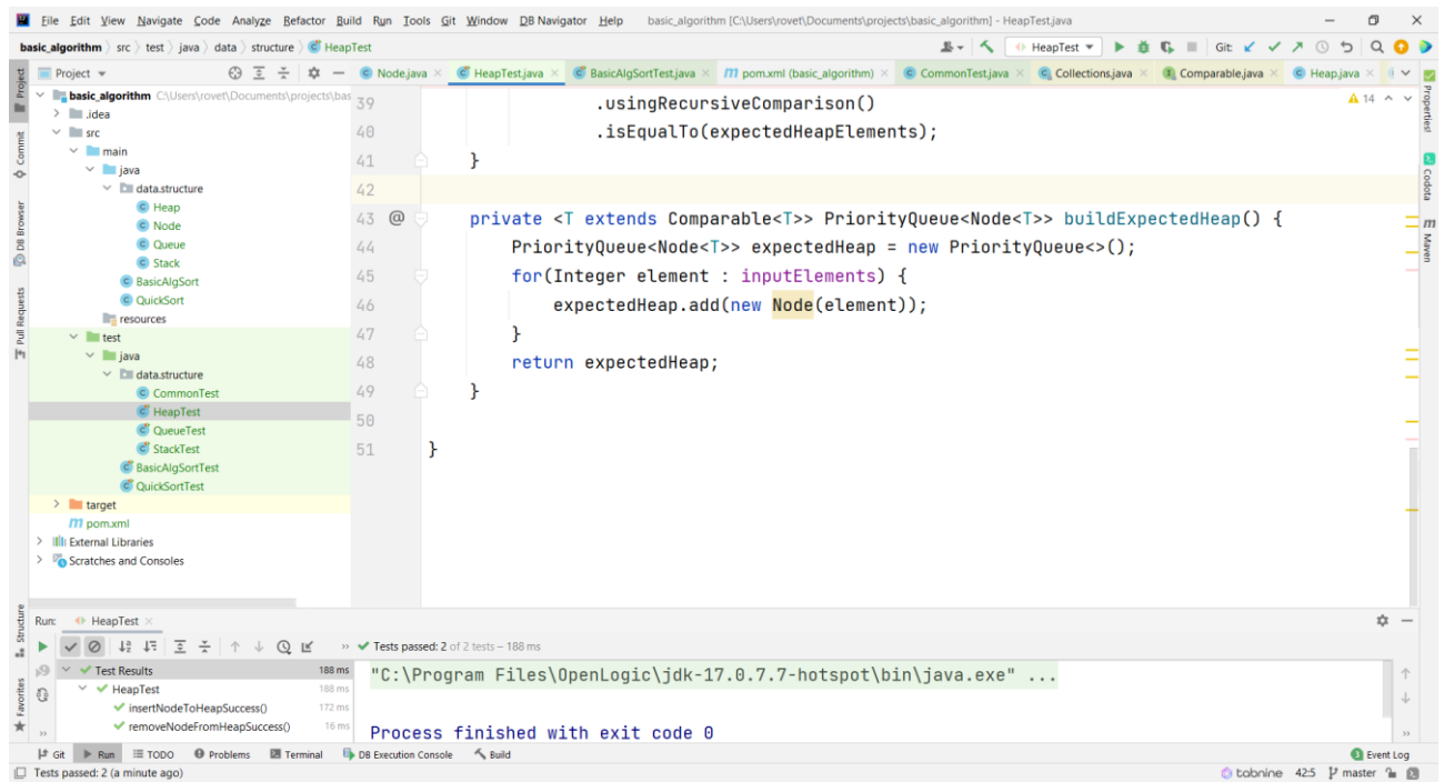
Рис.2. Тестування реалізації структури даних піраміди (а, б, в, г)
