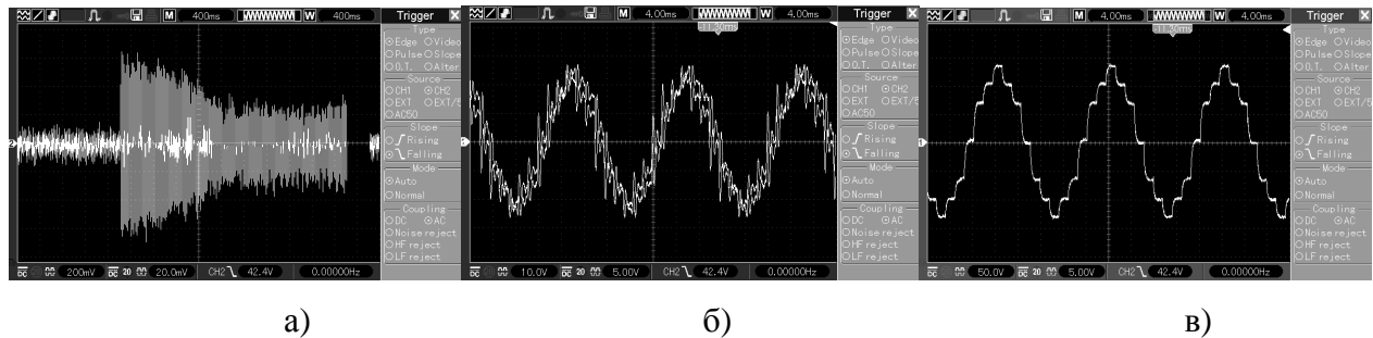
Рис.7. Результати досліджень на фізичній моделі: а) залежності струму статора при пуску від АБ, б) форма струму і напруги АД при живленні від АБ в усталеному режимі, в) форма напруги живлення АД від АБ
