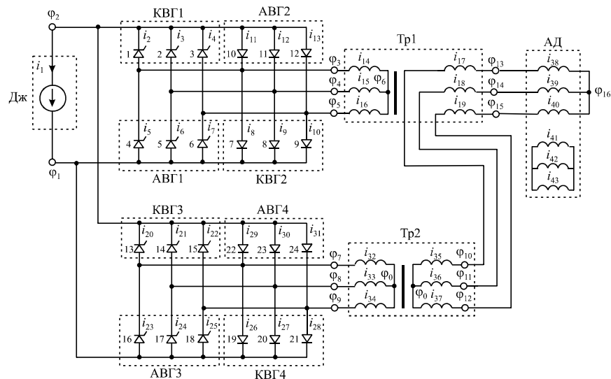
Рис.3. Розрахункова схема автономного джерела живлення АД системи внутрішнього протипожежного водопостачання
