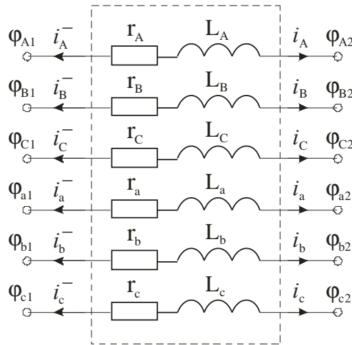
Рис.2. Розрахункова схема АД
