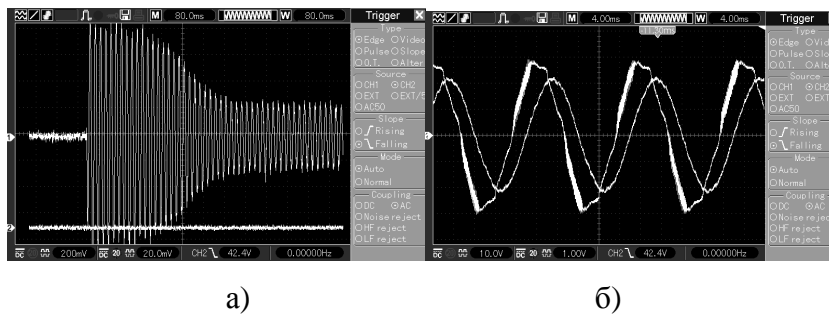
Рис.6. Результати досліджень при живленні АД від мережі: а) залежність струму статора при пуску, б) форма струму і напруги в усталеному режимі
