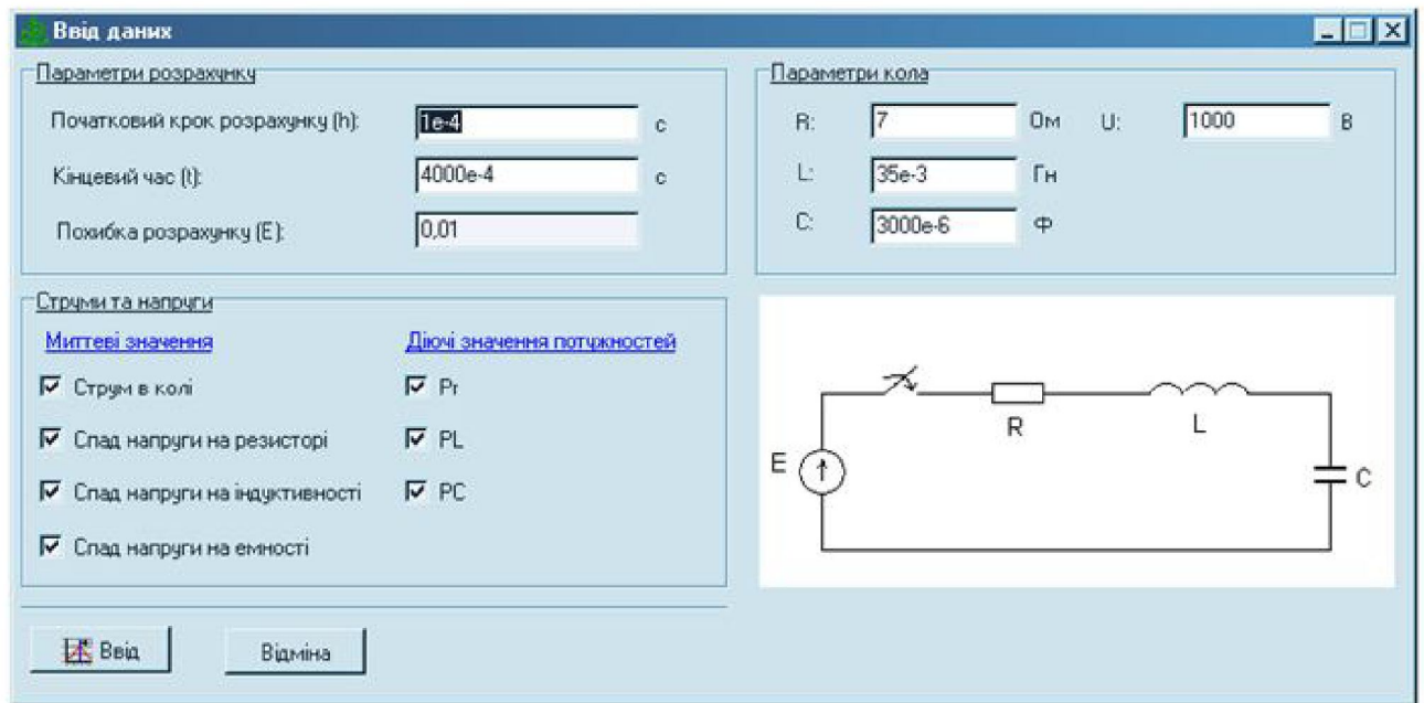
Рис. 2. Діалогове вікно вводу даних лабораторної роботи
