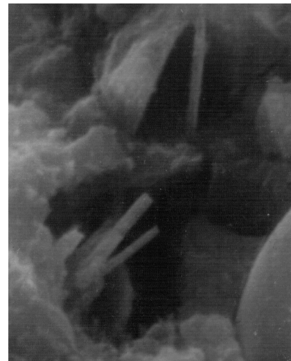
Рис. 2. Мікроструктура каменю на основі портландцементу ПЦ І-500, гідратованого 7 діб
