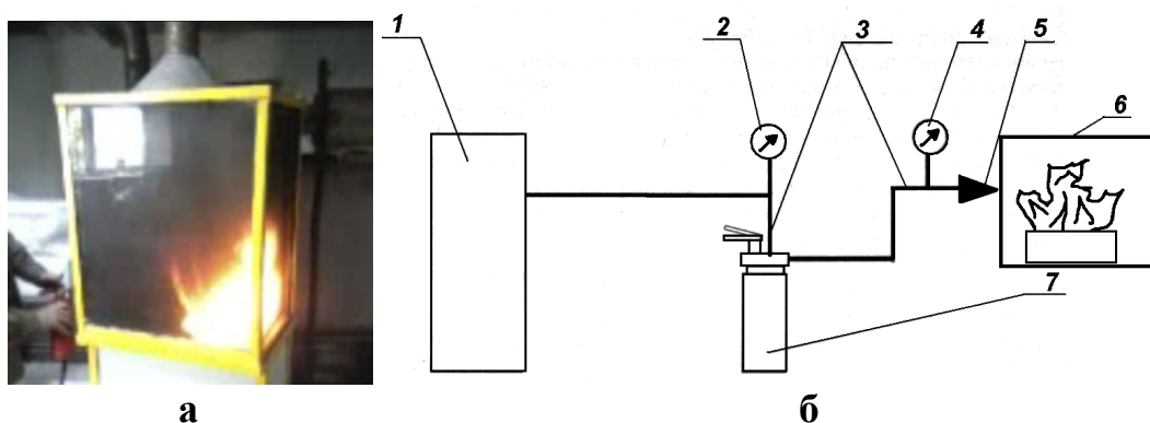
Рис. 1 – а – загальний вигляд спеціальної випробувальної камери зі скляною вітриною; б – схема установки для вогнегасних випробувань: 1 – балон із стисненим повітрям; 2, 4 – манометри; 3 – з'єднувальний шланг; 5 – центробіжна шнекова форсунка; 6 – осередок займання (вогнище класу В1), 7 – пристрій подачі ВВР типу вогнегасника ВВ-5
