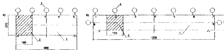
Рис. 1. Схема создания одностороннего (а) и локального (б) изменения объема материала. 1 – образцы; 2 – зона увлажнения; 3 – микроиндикатор часового типа
