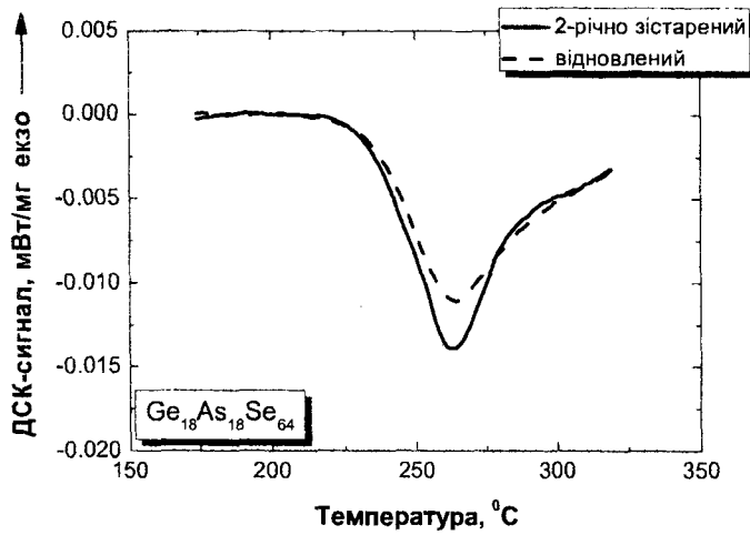
Рис. 1. ДСК-криві дворічно зістарених та відновлених ХС \text{Ge}_{18}\text{As}_{18}\text{Se}_{64} .
