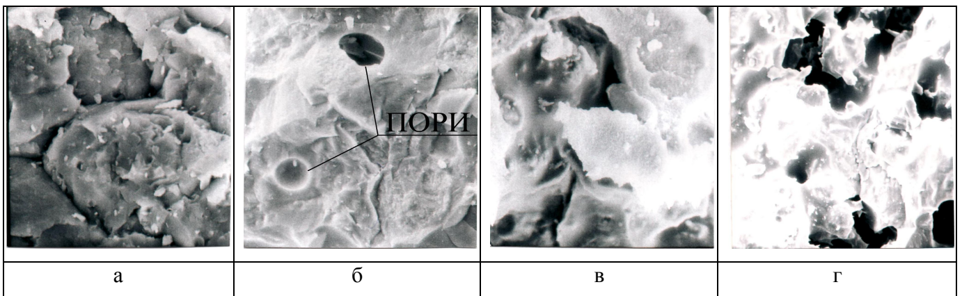
Рис. 2. Зміна мікроструктури захисного покриття при нагріванні:
