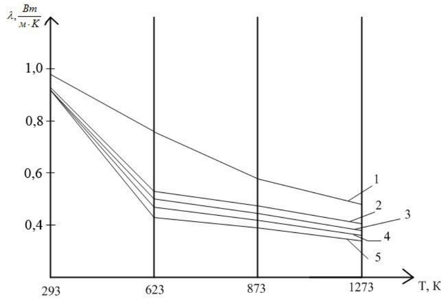
Рис. 1. Залежність коефіцієнта теплопровідності вогнезахисного бетону при нагріванні:
