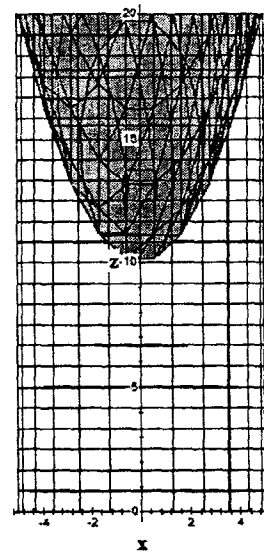
Рис. 2. Форма рідини в циліндрі при його швидкості обертання: а) \omega = 1 рад/с, б) \omega = 2 рад/с
