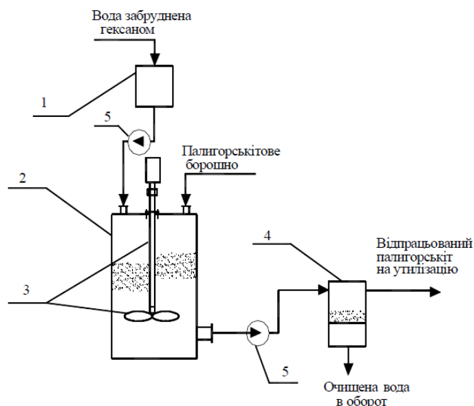
Рис. 1. Технологічна схема очищення стічних вод від гексану:
