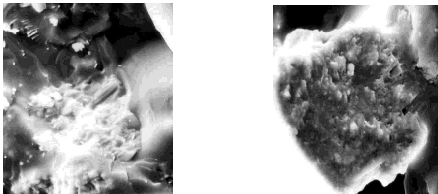
Рис.2. Зміна мікроструктури покриттів на основі композиції KO-08 - Al_2O_3 - TiO_2 з додатком Cr_2O_3 при нагріванні до 973 К
