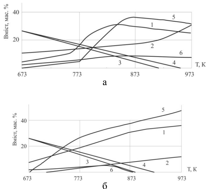
Рис.1 Зміна фазового складу покриття на основі наповнених оксидом алюмінію титану поліметилфенілсилоксану в процесі нагрівання : 1 – муліт; 2 – скловидна фаза; 3 – оксид алюмінію; 4 – оксид титану; 5 – тіаліт; 6 – кристобаліт (а - зі скловидним додатком, б – з додатком Cr_2O_3 )
