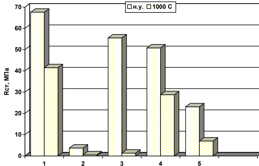
Рис. 1. Міцність цементних мінералів у віці 28 днів при нагріванні до 1200 0 С:
