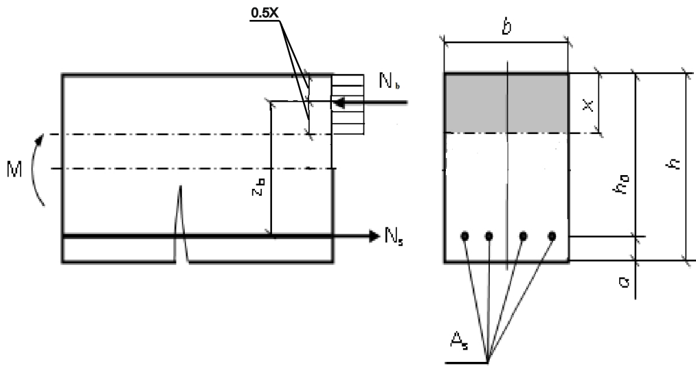
Рис. 1. Розрахункова модель напружено-деформованого стану залізобетону при згині
