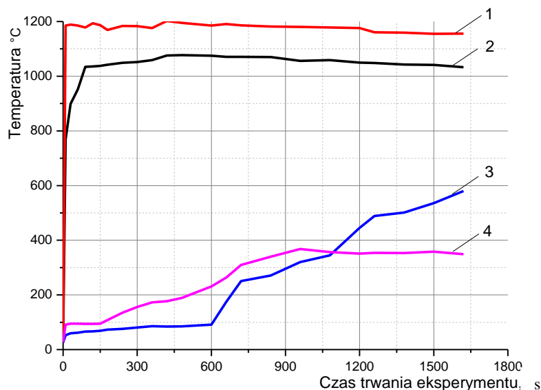
Rys. 2. Charakterystyka wzrostu temperatury w czasie oddziaływania płomienia na elementy konstrukcyjne: 1 – temperatura płomienia, [°C]; 2 - temperatura ściany po stronie ogrzewanej[°C]; 3 – temperatura ściany po stronie nieogrzewanej[°C]; 4 - temperatura w środku konstrukcji, [°C].
